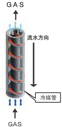
ZC-100 \alpha /200 \alpha 用 高性能二重構造小型熱交換器
